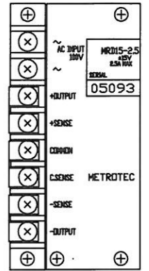
MRD15用 入出力表示図
