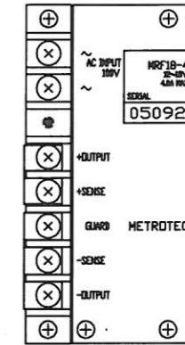
MRFシリーズ 入出力表示図
